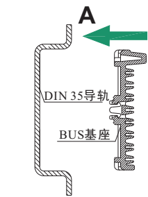
A. 将BUS基座卡装到DIN 35导轨上；
