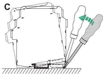
C. 用螺丝刀在卡件处按箭头所示方向稍微撬起安全栅，从而向下牵动弹簧销，旋转安全栅。
