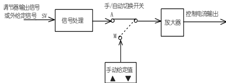
Q型手操器控制原理图
