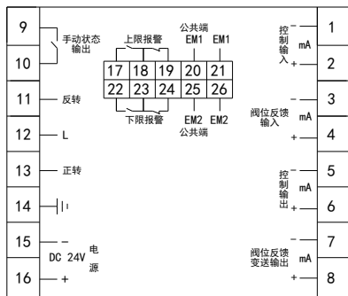
直流24V 供电
