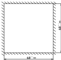
仪表盘开孔尺寸
