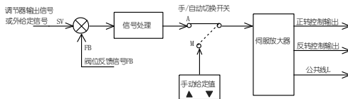
D型手操器控制原理图
