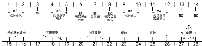
交流 220V 供电
