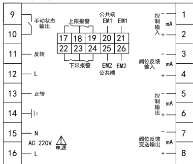
交流220V 供电
