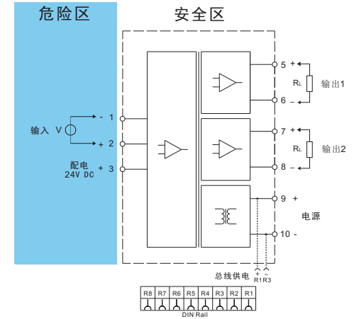
单入双出接线图
