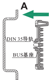
A. 将BUS底座卡装到DIN 35导轨上；
