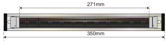
NPPB-DIN350尺寸
