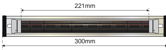
NPPB-DIN300尺寸
