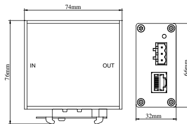
外形尺寸
