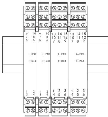
水平安装示意图
