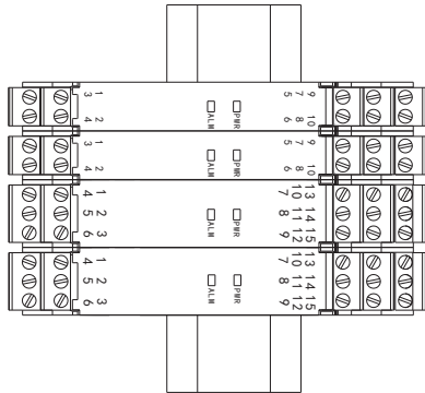
垂直安装示意图
