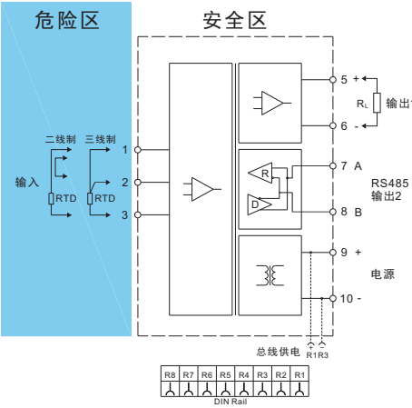
单路电流/电压输出，单路RS485输出接线图
